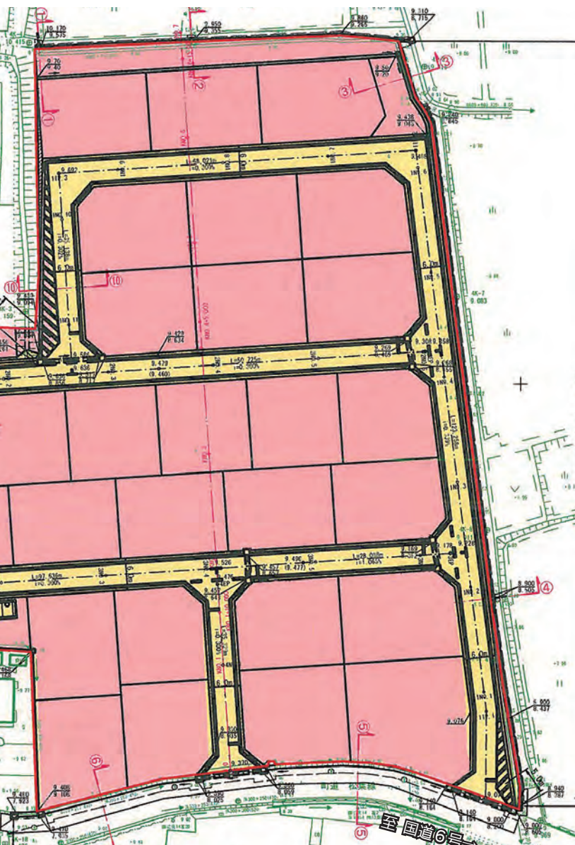
造成計画平面図（広野町下北迫地区）
